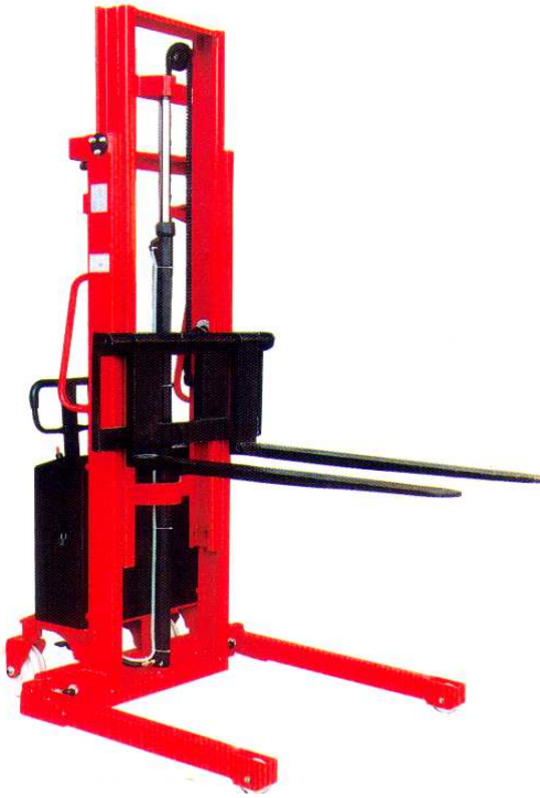
HES-160S avec longerons encadrant et fourches réglable (sur commande)
